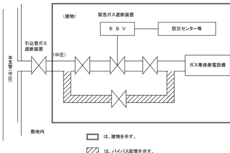
緊急ガス遮断装置のバイパス配管
