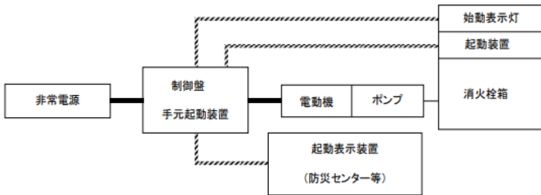
屋外消火栓設備の非常電源回路等
