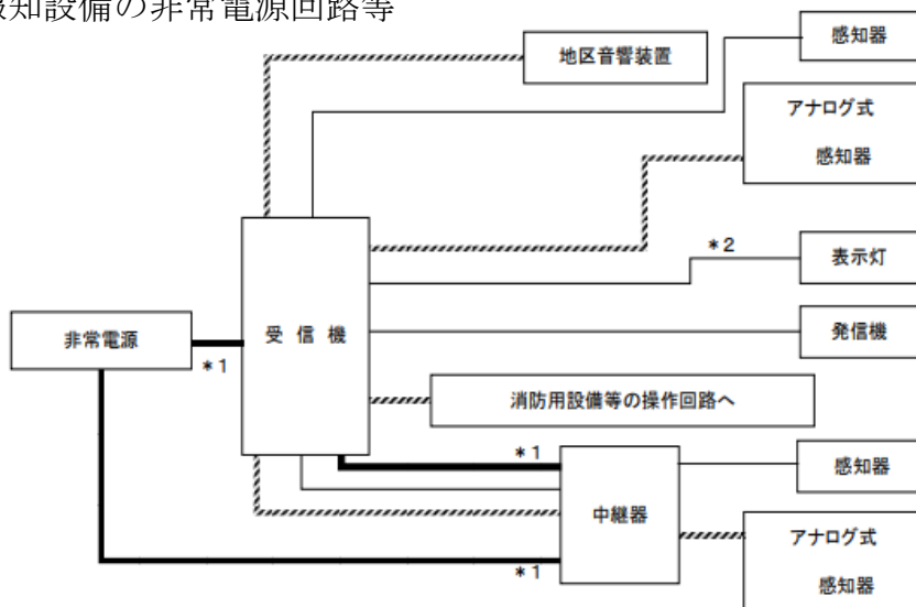
自動火災報知設備の非常電源回路等
